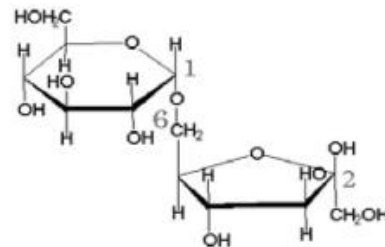
그림 1. 팔라티노스의 화학구조식
